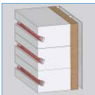
3-vrstvá vyzdívka stěn série KE-L a KE-N
