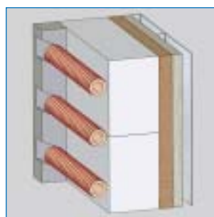
4-vrstvá vyzdívka stěn série KE-S/S+/SH
